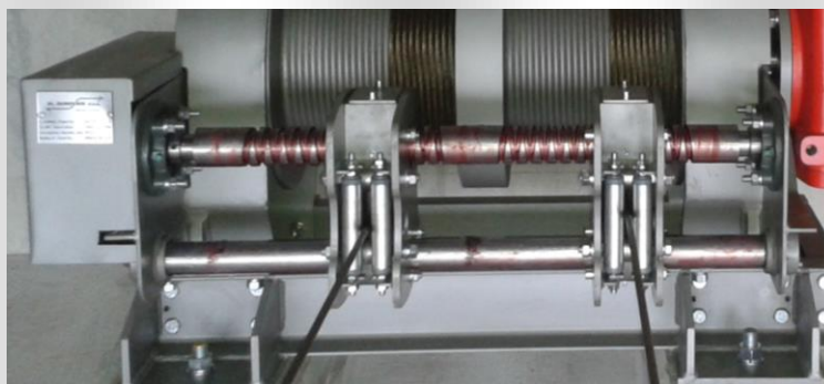
Sistem samodejnega navijanja jeklene vrvi na boben.
